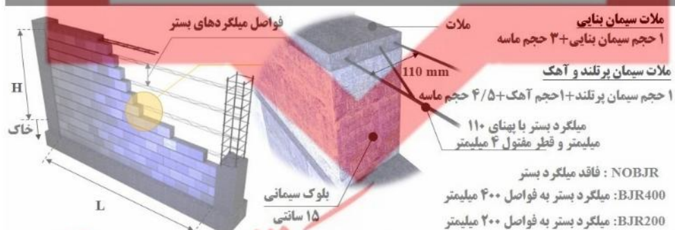
شکل (۴-۱). ظرفیت خارج از صفحه پانل بنایی ۱۵ سانتی ساخته شده از بلوک‌های سیمانی توخالی
